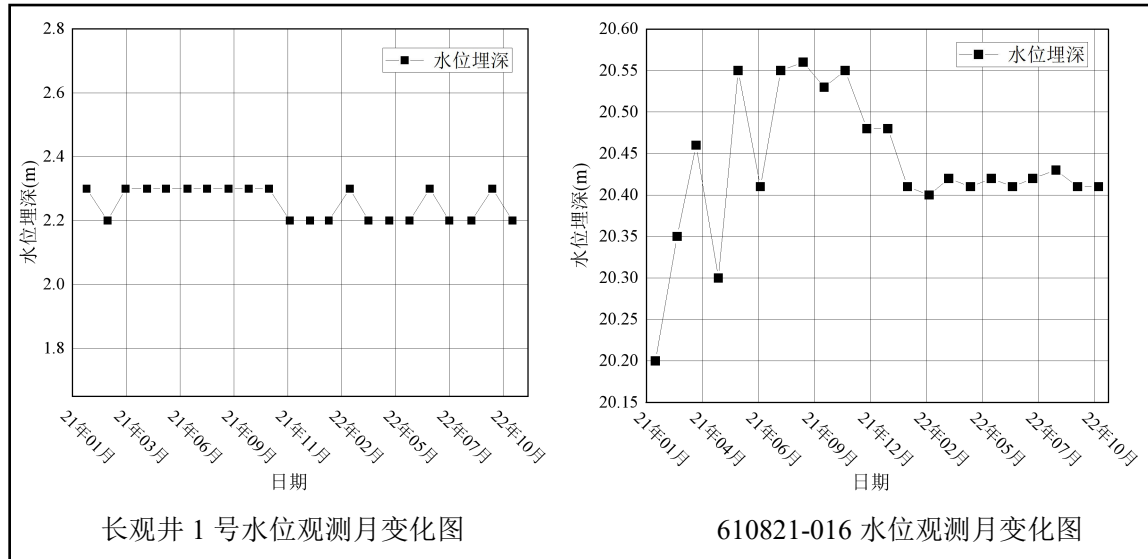
图 4.2.1-2 井田长观孔水位月变化图
